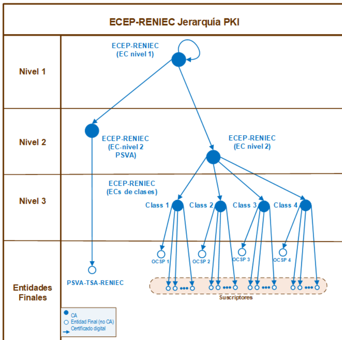
Figura 1: Diagrama de la jerarquía PKI del RENIEC
