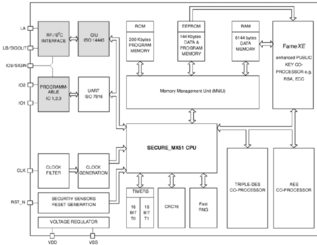
Figura 1 - Diagrama de bloques del Controlador NXP P5CD144V0B para Tarjeta Inteligente (NXP Semiconductors)
