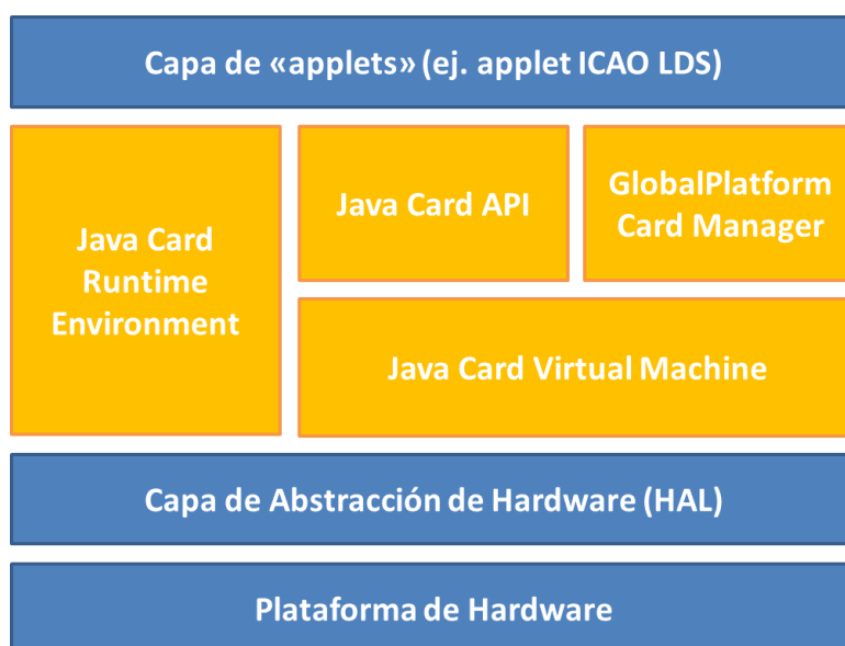
Figura 4 - Componentes JavaCard en el sistema operativo del DNle
