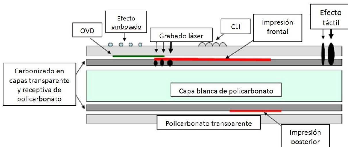
Figura 8 - Estructura de capas de policarbonato de la tarjeta del DNle
