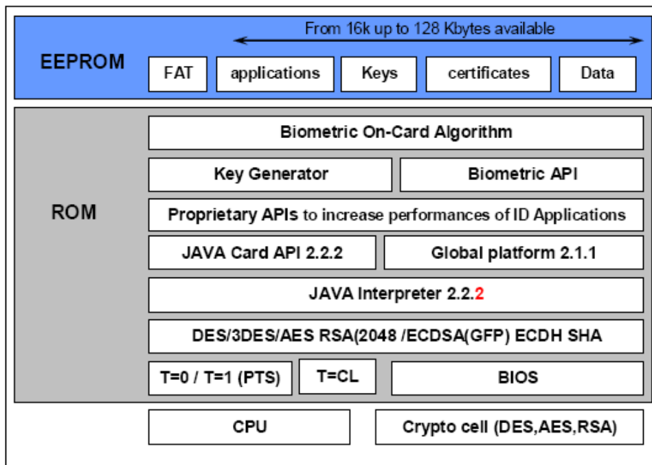
Figura 2 - Diagrama de bloques lógico del sistema operativo ID-One-Cosmo-V7 (Oberthur Technologies)
